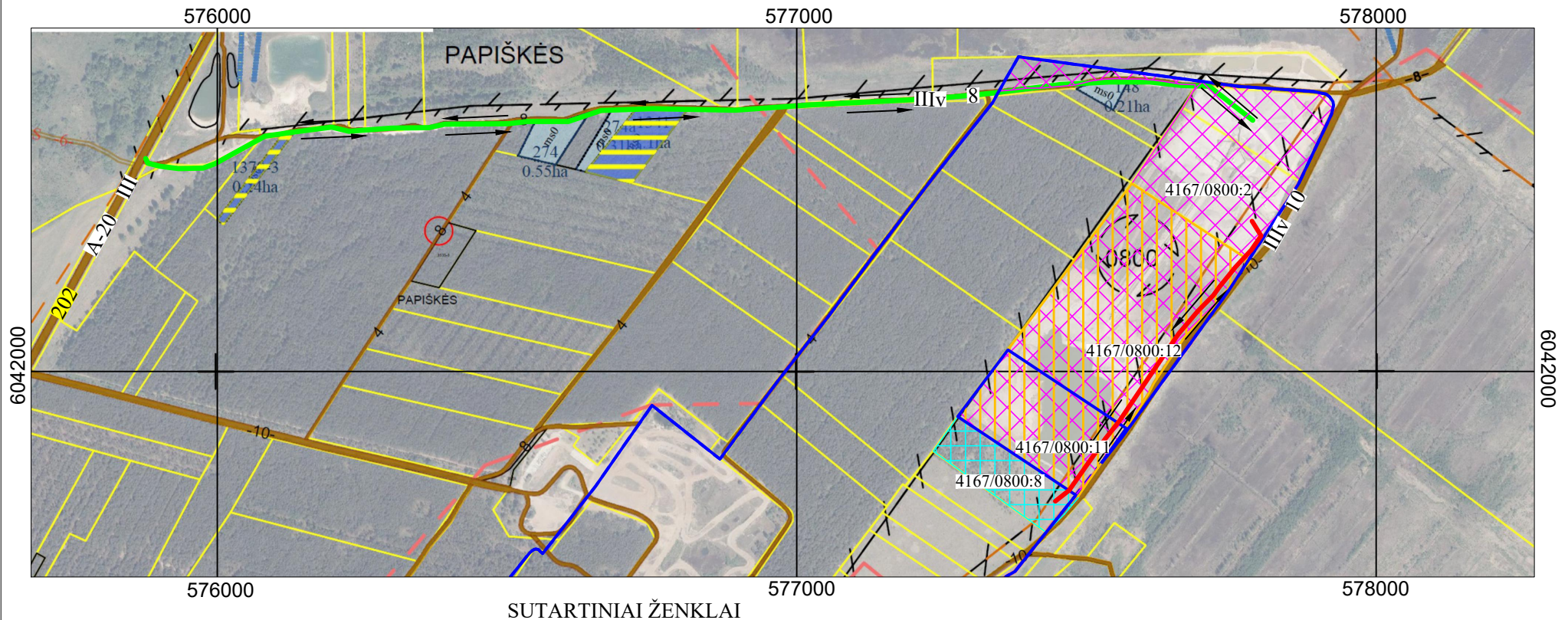
2.6 pav. Papiškių smėlio ir žvyro telkinio dalies susisiekimo schema, M 1:10 000
